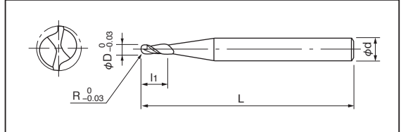
材質: DZコート(TiAIN系)
