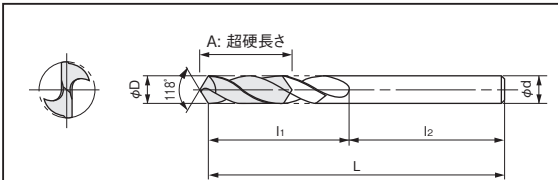
材種：ノンコート超硬K種
